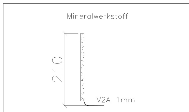
Seitenschnitt
