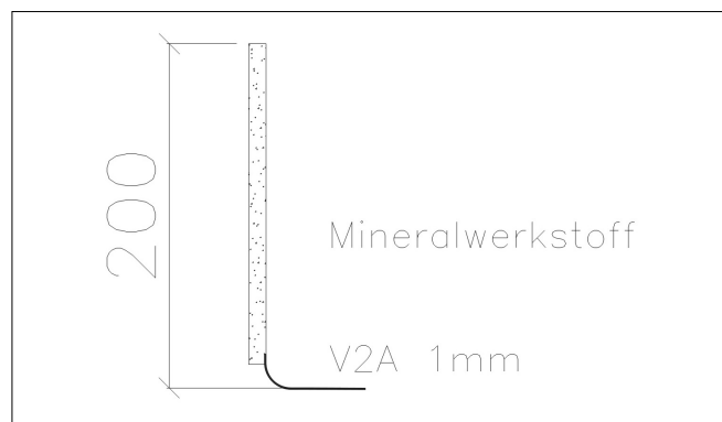
Seitenschnitt
