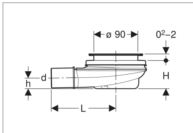
Seitenschnitt
