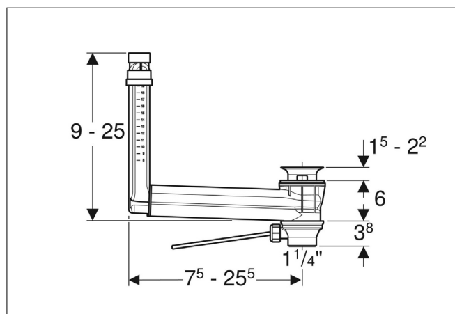
Seitenschnitt
