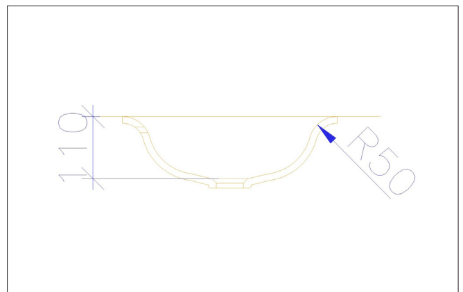
Seitenschnitt
